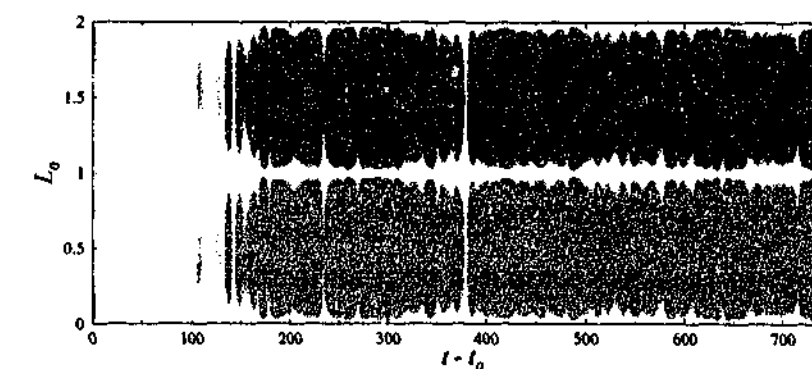
(d) Re = 280, \lambda_d = 2L_0 .
