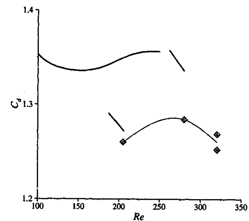
(a) Total drag ( C_d ).
